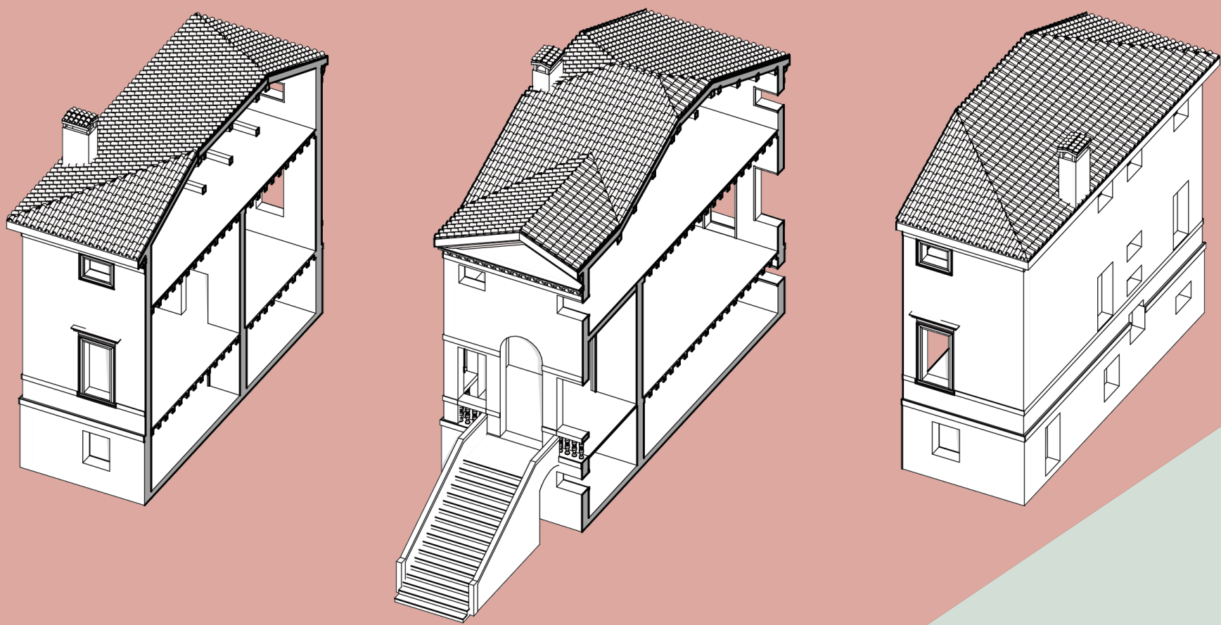
SPACCATO LONGITUDINALE DEI TRE PIANI SCALA 1:200
