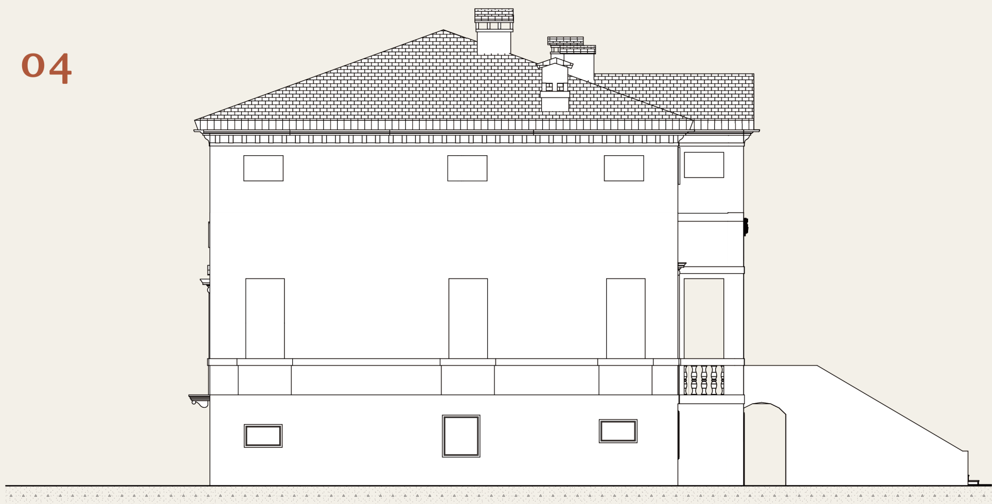
PROSPETTO OVEST
