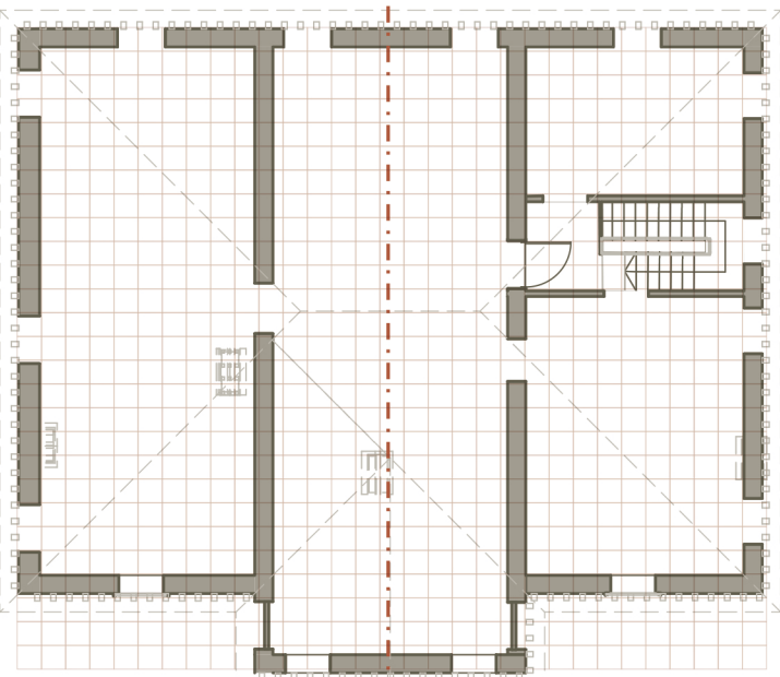
III PIANO SOTTOTETTO
