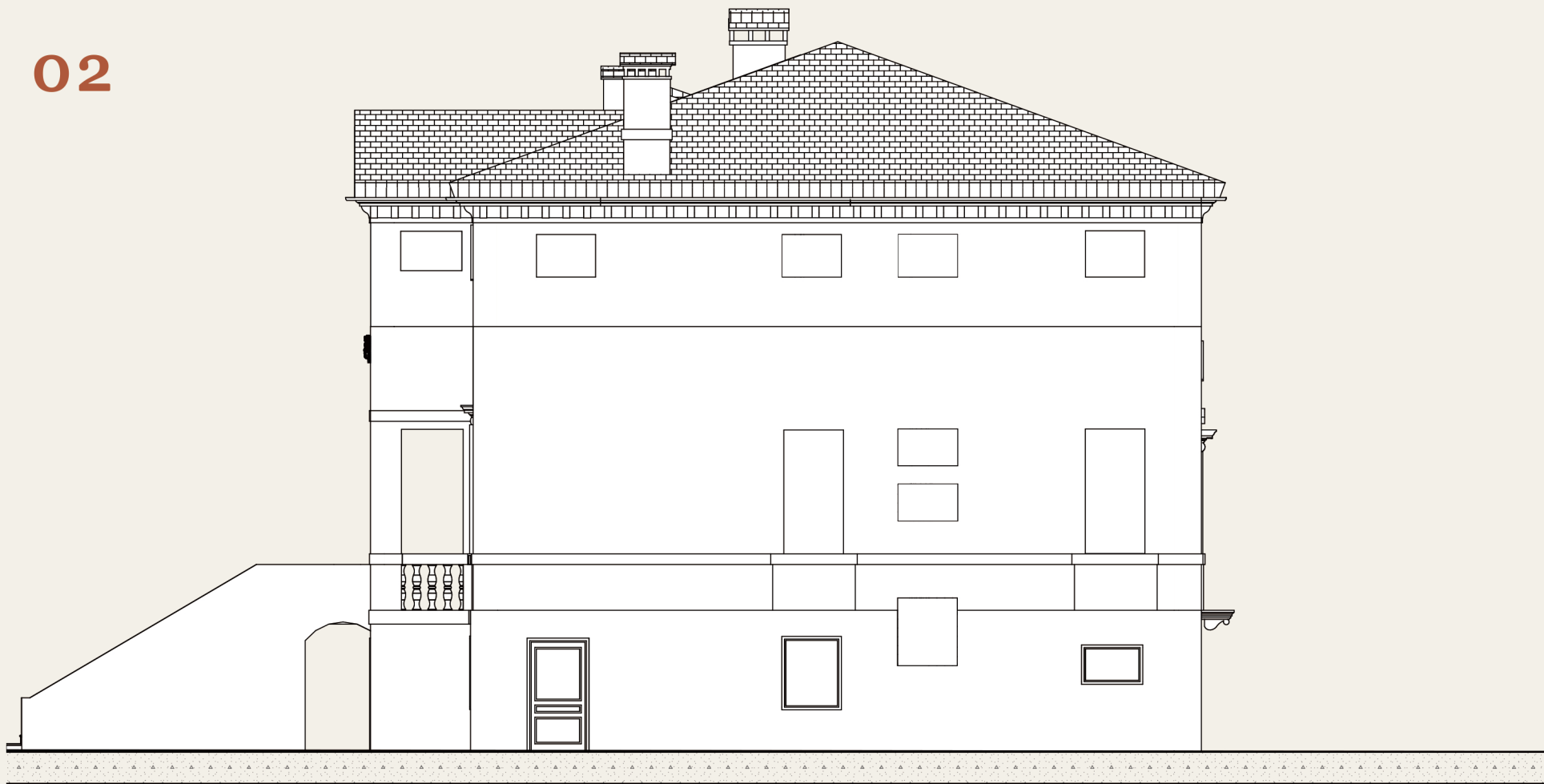
PROSPETTO EST
