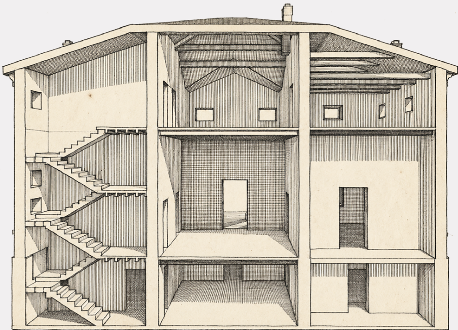
VISTA PROSPETTICA 3D. SEZIONE NORD
