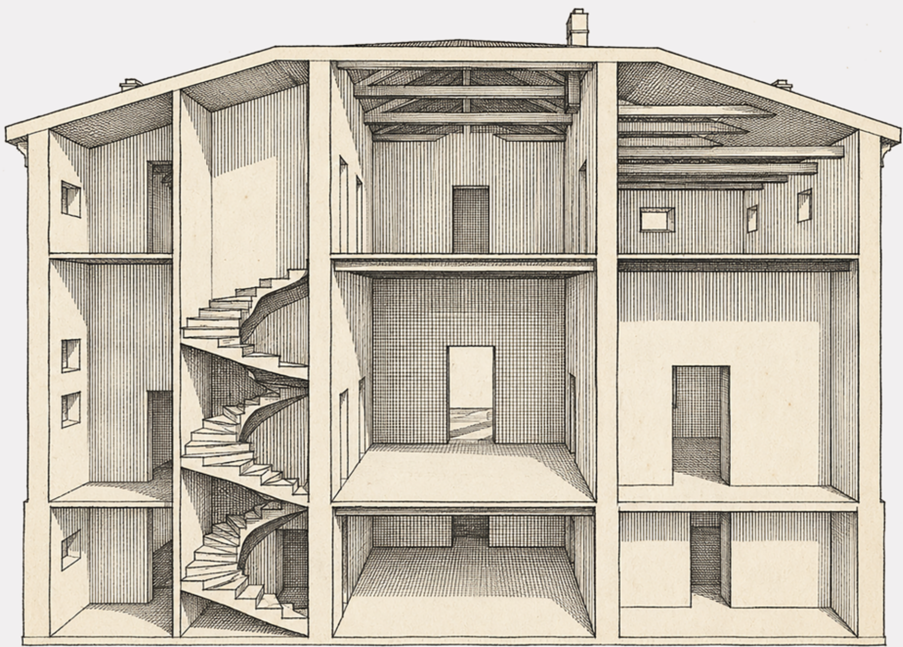
VISTA PROSPETTICA 3D. SEZIONE NORD
