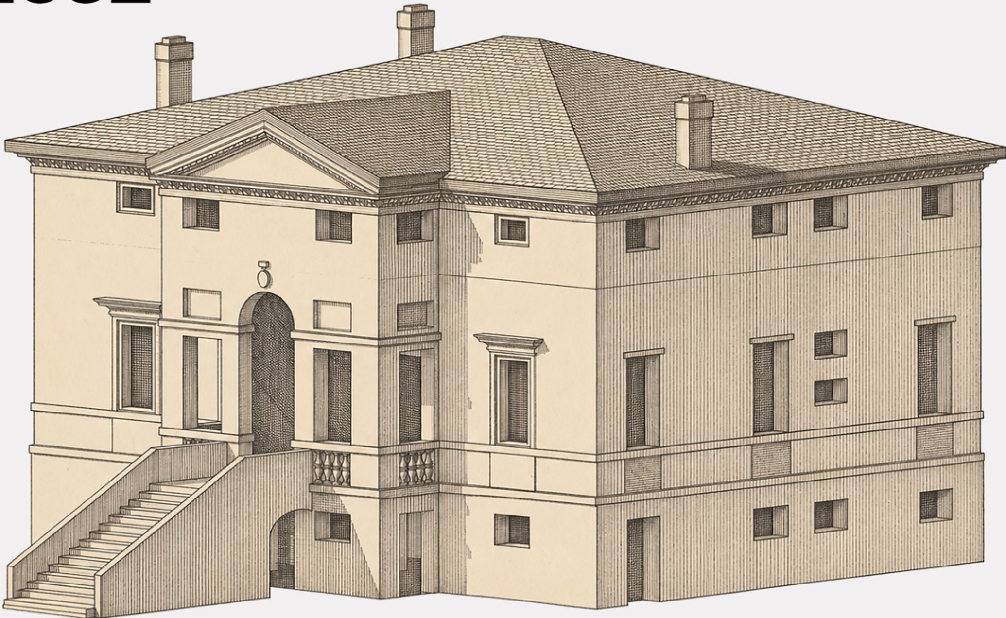
VISTA ASSONOMETRICA 3D. SPIGOLO SUD-EST
