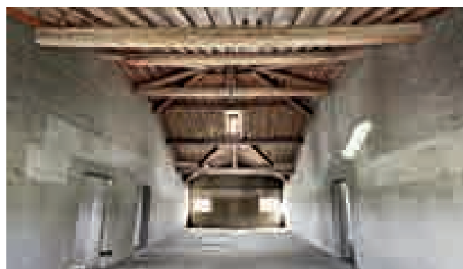
41 Viste del salone centrale al piano nobile, e della stanza principale al piano sottotetto, nel modello 3D realizzato da Paolo Mazzuccato 41 Views of the central hall on the piano nobile and the main room in the attic, from the 3D model made by Paolo Mazzuccato
