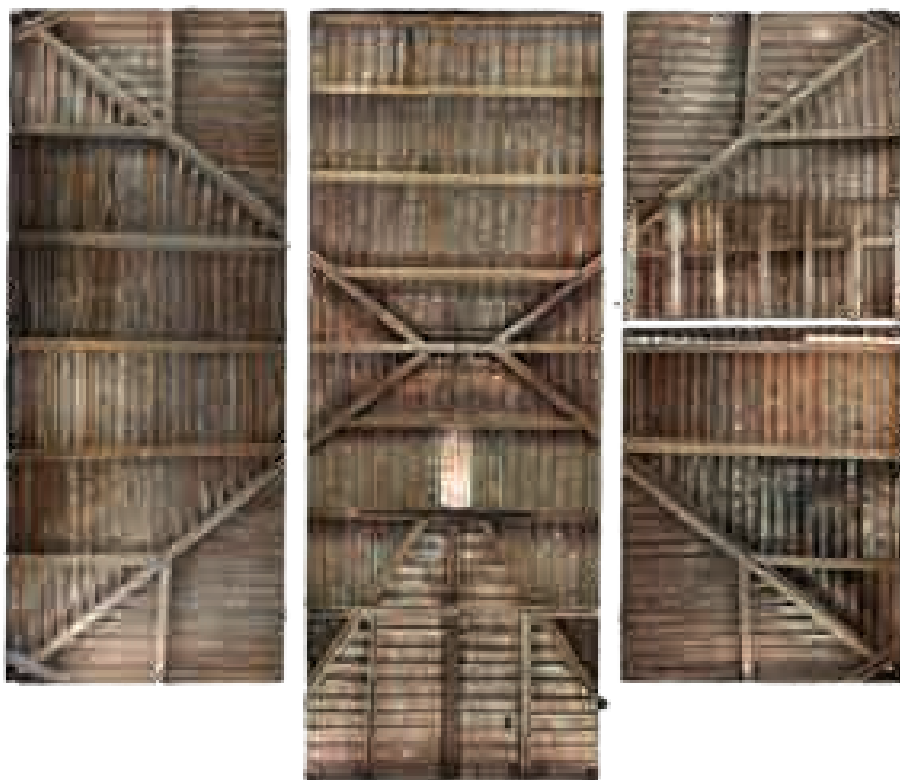
46 Rilievo fotogrammetrico della copertura di Villa Forni Cerato, effettuata dal Politecnico di Milano nel 2018 46 Photogrammetric relief of the roofing of Villa Forni Cerato, performed by the Politecnico di Milano in 2018
