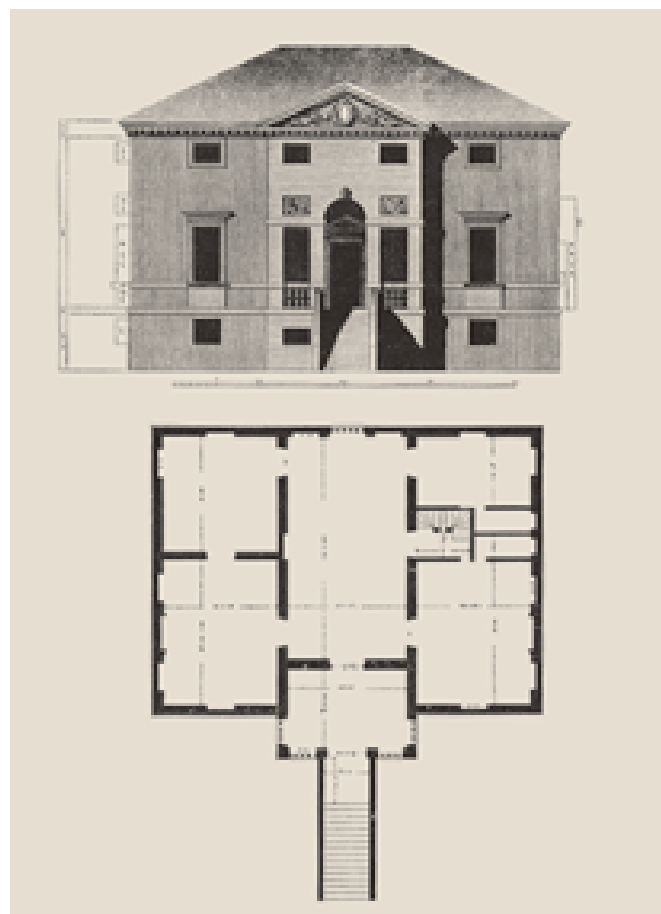
43 Rilievi storici di Villa Forni Cerato a Montecchio Precalcino del prospetto e del piano nobile con accesso da sud.
